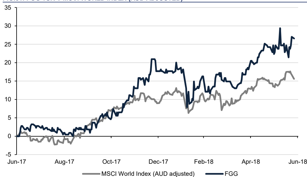
FIG.51: FGG TSR V MSCI WORLD INDEX (AUD ADJUSTED)
